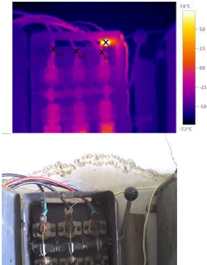
Термограмма 2.1.4.14 Температурное поле электропроводящих частей вводного рубильника скважины №3827
